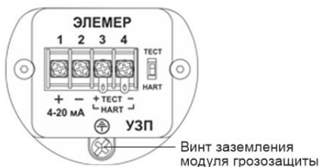
Рисунок 2.4 - Внешний вид коммутационной платы и функциональное расположение контактов для корпуса АГ-03, НГ-03 (АИР-20/М2-Н-ГС со встроенным модулем грозозащиты)
