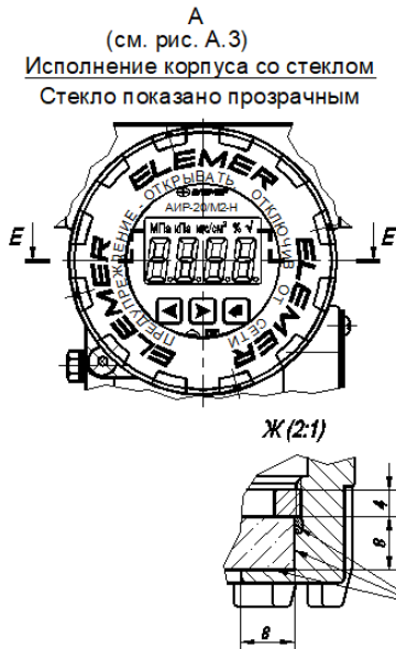
Чертеж средств взрывозащиты. Рисунок А.5
