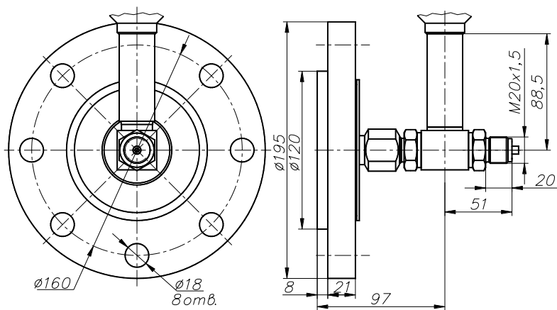
Модели 620, 640
