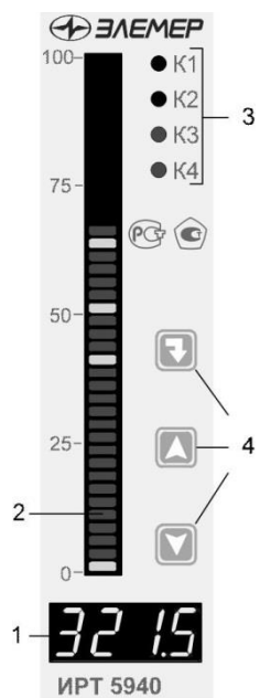
Рисунок 2.3 – Передняя панель ИРТ 5940/М2
