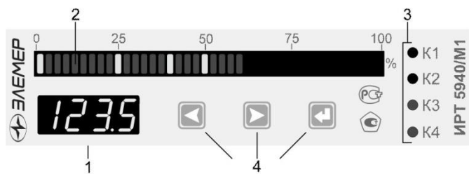
Рисунок 2.2 – Передняя панель ИРТ 5940/М1
