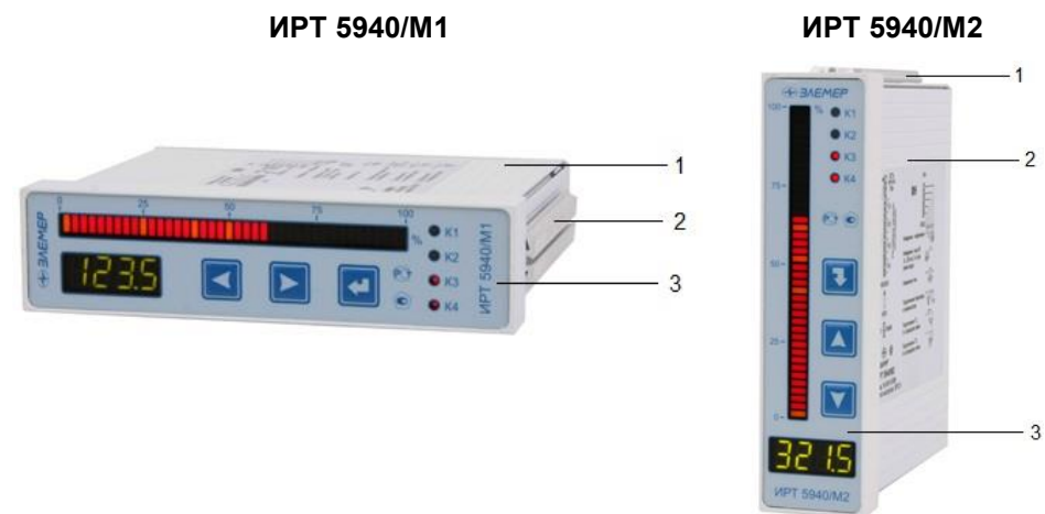
Рисунок 2.1 – Общий вид ИРТ
