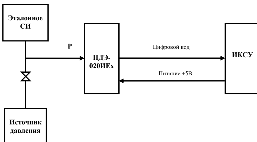
Рисунок А.2 – При подключении преобразователя к ИКСУ
