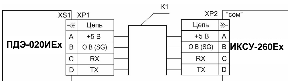
Рисунок 4 – Схема внешних электрических подключений преобразователя к ИКСУ-260Ех
