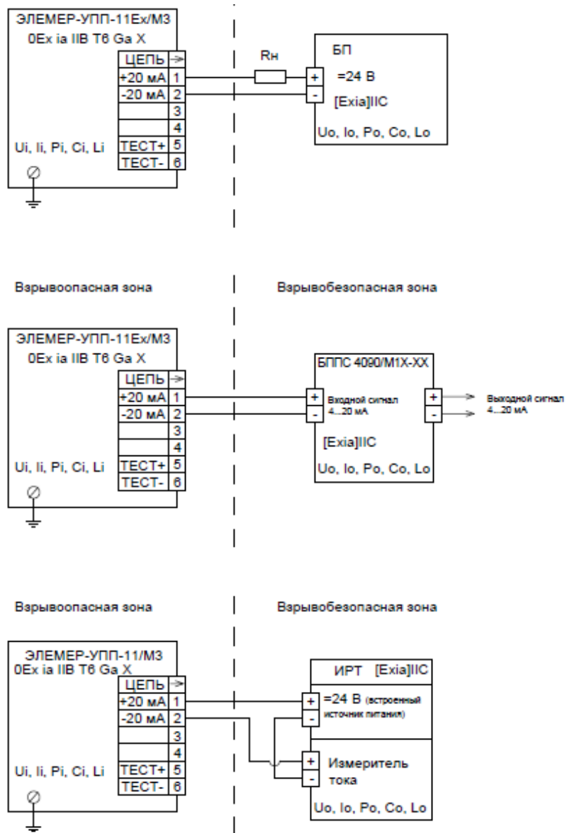
Рисунок Б.2 – Схема электрическая подключений УПП-11Ех/М3 через кабельный ввод Продолжение приложения Б
