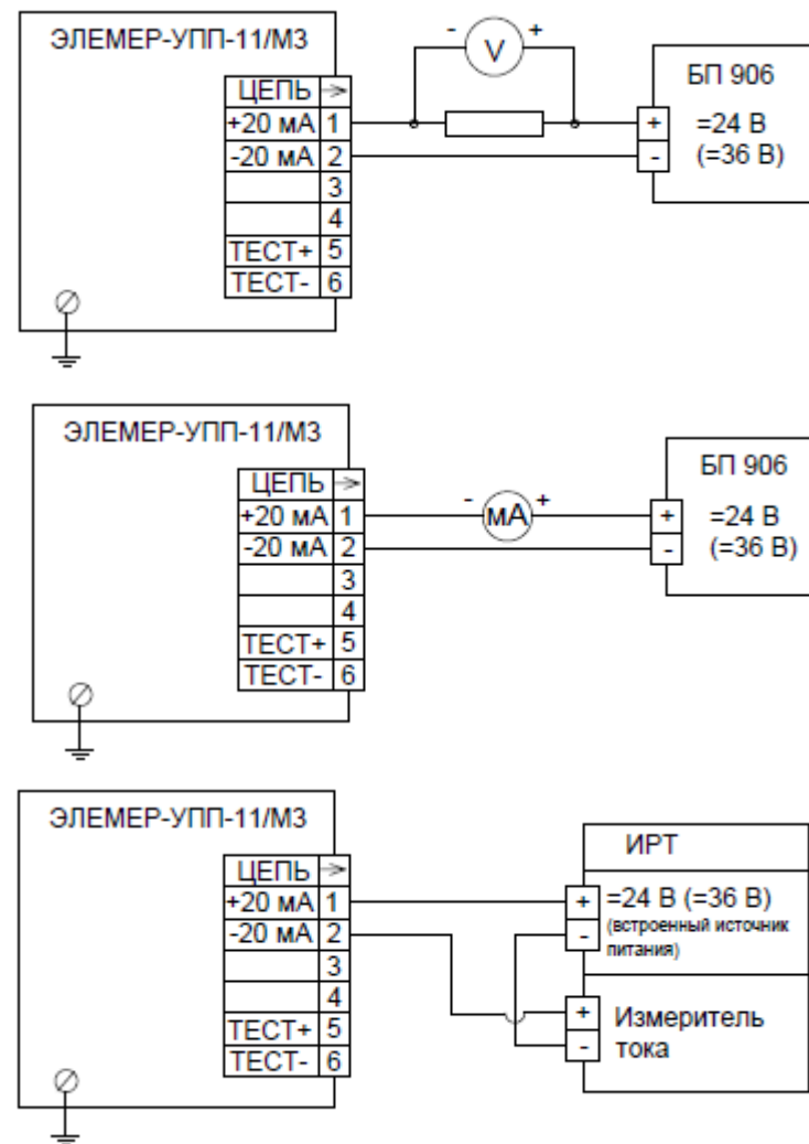
Рисунок Б.1 – Схема электрическая подключений УПП-11/М3 и УПП-11Exd/М3 через кабельный ввод
