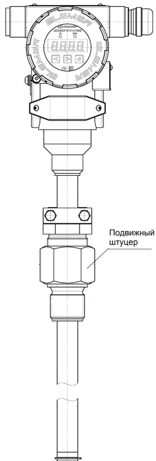
Рисунок В.2 – УПП-11/М3 с подвижным штуцером, индекс заказа «-»
