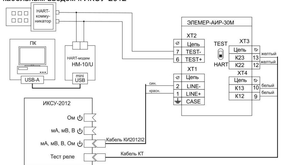
Рисунок 3.1.2 - Схема электрическая подключений ЭЛЕМЕР-АИР-30М с выходным сигналом 4-20 мА с каналами сигнализации на электромагнитных реле с кабельным вводом к ИКСУ-2012
