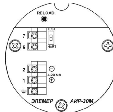
Рисунок 2.4 - Модуль подключений АИР-30М с выходным сигналом 4-20 мА без реле
