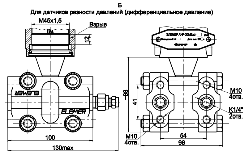
Рисунок А.13 - Чертеж средств взрывозащиты
