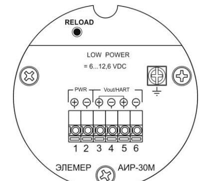
Рисунок 2.7 - Модуль подключений АИР-30М с выходными сигналами напряжения 0,8-3,2 В; 0,5-4,5 В; 1-5 В
