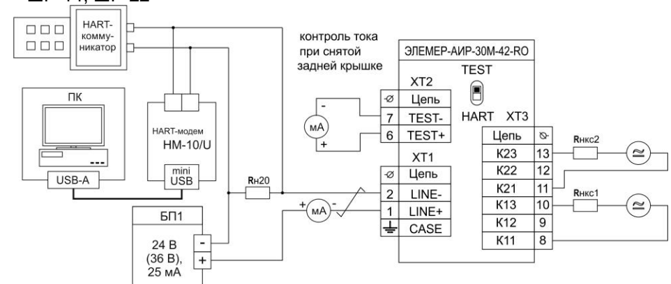
Рисунок 3.13 - Схема электрическая подключений ЭЛЕМЕР-АИР-30М с выходным сигналом 4-20 мА с каналами сигнализации на оптореле с кабельными вводами
