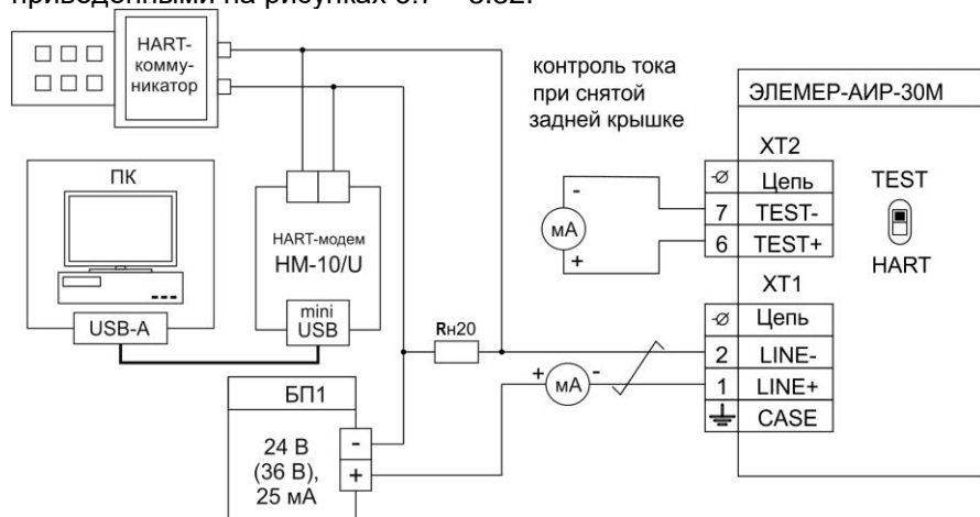
Рисунок 3.7 - Схема электрической подключений ЭЛЕМЕР-АИР-30М с выходным сигналом 4-20 мА без каналов сигнализации с кабельным вводом
