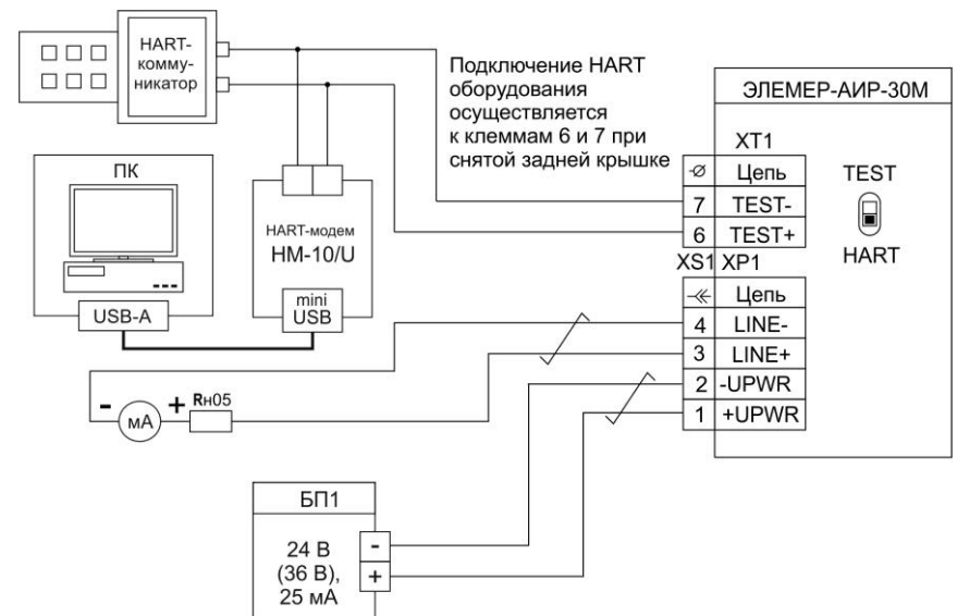
Рисунок 3.12 - Схема электрическая подключений ЭЛЕМЕР-АИР-30М с выходным сигналом 0-5 мА без каналов сигнализации с разъемами ШР-14, ШР-22
