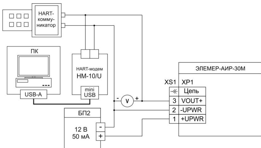
Рисунок 3.10 - Схема электрическая подключений ЭЛЕМЕР-АИР-30М с выходными сигналами напряжения 0,8-3,2 В; 0,5-4,5 В; 1-5 В с разъемами ШР14, ШР22
