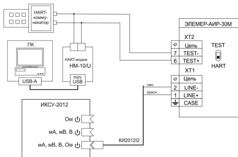
Рисунок 3.1 - Схема электрических подключений ЭЛЕМЕР-АИР-30М с выходным сигналом 4-20 мА без каналов сигнализации с кабельным вводом к ИКСУ-2012
