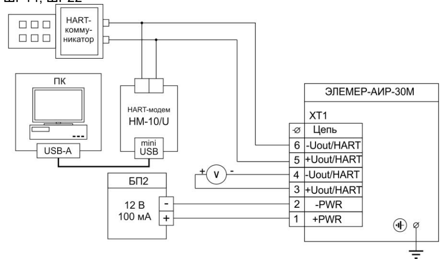
Рисунок 3.9 - Схема электрическая подключений ЭЛЕМЕР-АИР-30М с выходными сигналами напряжения 0,8-3,2 В; 0,5-4,5 В; 1-5 В с кабельным вводом
