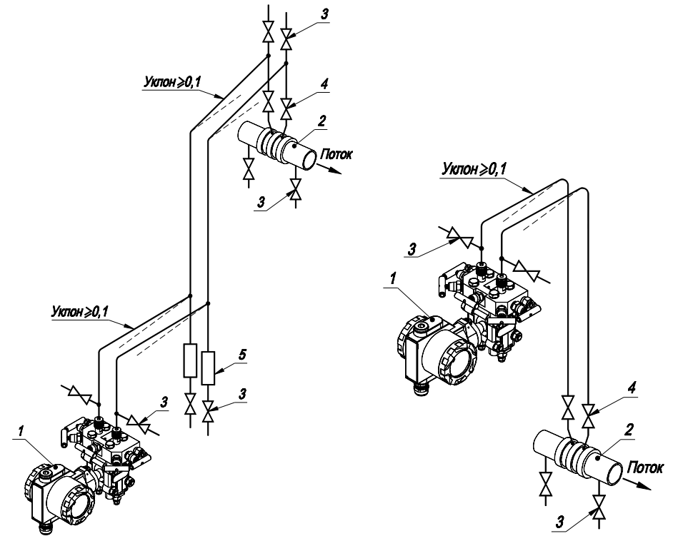
а) АИР-30М ниже сужающего устройства б) АИР-30М выше сужающего устройства
