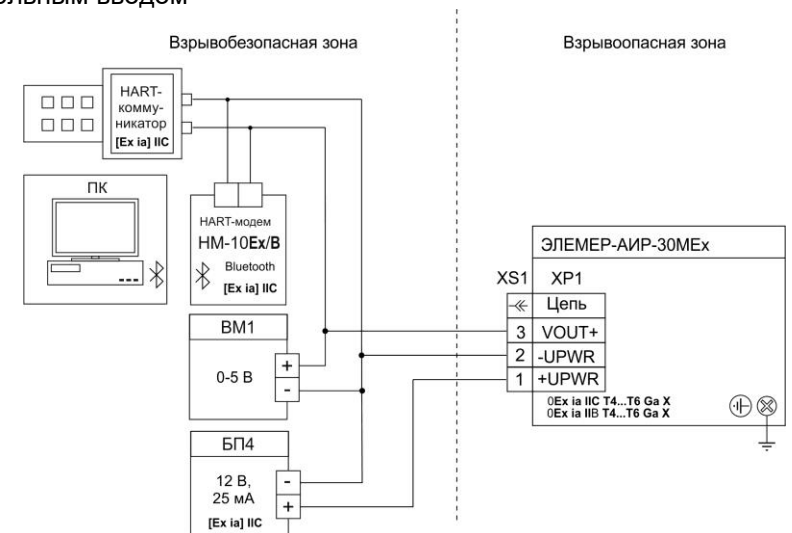
Рисунок 3.32 - Схема электрическая подключений ЭЛЕМЕР-АИР-30МEx с выходными сигналами напряжения 0,8-3,2 В; 0,5-4,5 В; 1-5 В с разъемами ШР-14, ШР-22
