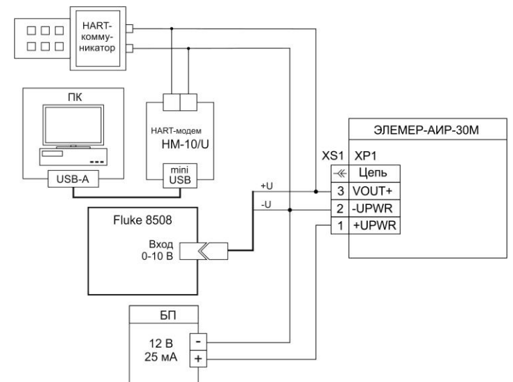
Рисунок 3.6 - Схема электрическая подключений ЭЛЕМЕР-АИР-30М с выходными сигналами напряжения 0,8-3,2 В; 0,5-4,5 В; 1-5 В с разъемами ШР-14, ШР-22
