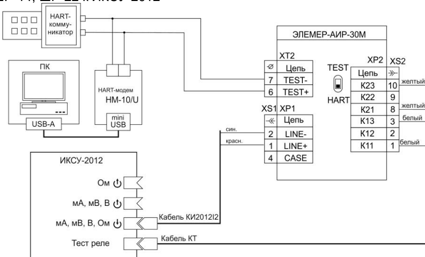
Рисунок 3.2.1 - Схема электрическая подключений ЭЛЕМЕР-АИР-30М с выходным сигналом 4-20 мА с каналами сигнализации на оптореле с разъемами ШР-14, ШР-22 к ИКСУ-20
