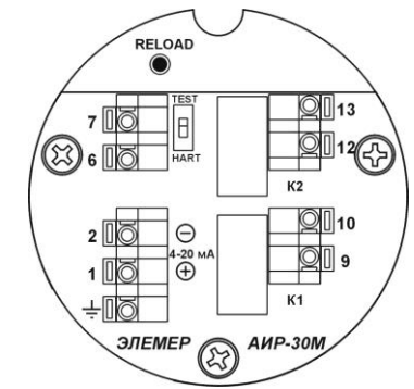
Рисунок 2.5 - Модуль подключений АИР-30М с выходным сигналом 4-20 мА и электромагнитными (поляризованными) реле
