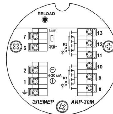
Рисунок 2.6 - Модуль подключений АИР-30М с выходным сигналом 4-20 мА и оптореле
