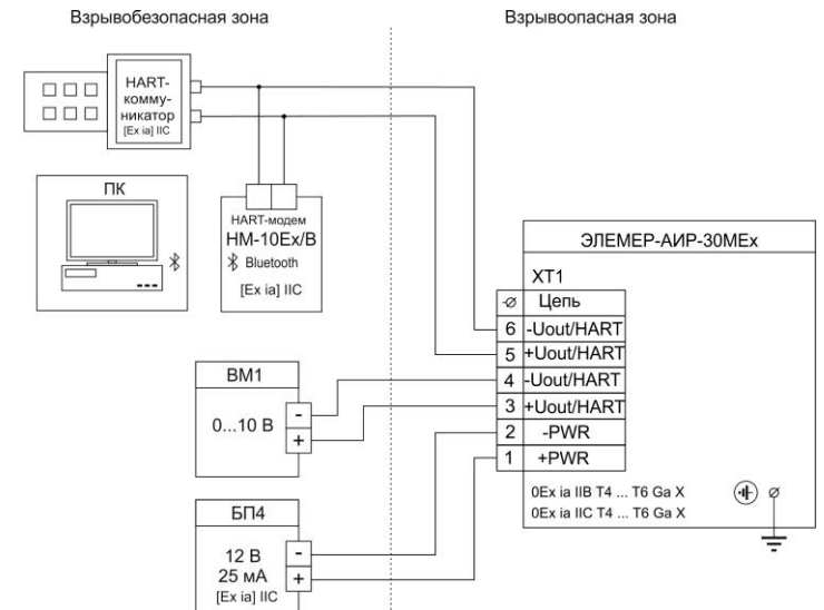
Рисунок 3.31 - Схема электрическая подключений ЭЛЕМЕР-АИР-30МEx с выходными сигналами напряжения 0,8-3,2 В; 0,5-4,5 В; 1-5 В с кабельным вводом
