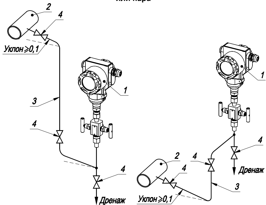
а) АИР-30М ниже точки отбора б) АИР-30М выше точки отбора
