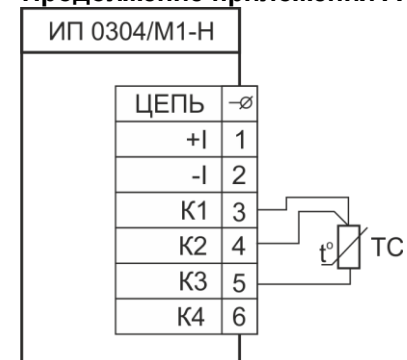
Рисунок А.3 – Подключение сопротивления к ИП 0304/М1-Н, трёхпроводная схема
