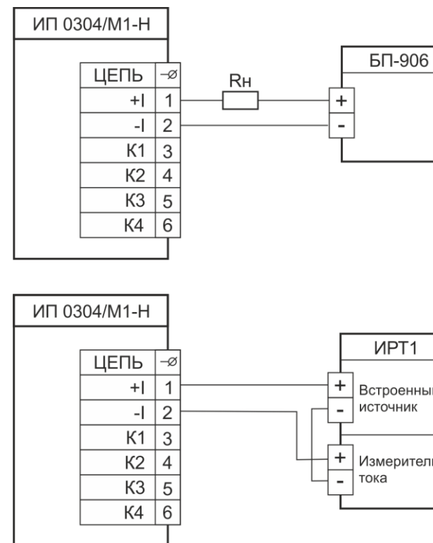
Рисунок А.4 - Схема электрическая подключений ИП 0304/М1-Н по унифицированному токовому сигналу 4...20 мА
