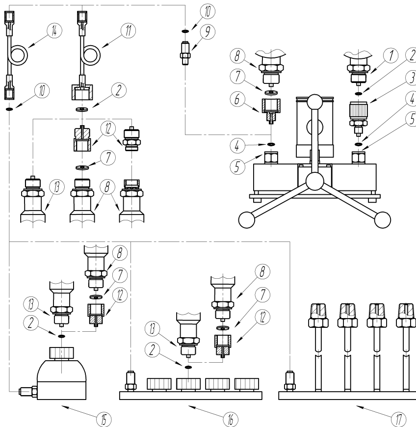
Рисунок А.1 Схема соединений для пресса гидравлического ручного «ЭЛЕМЕР-PR-1200»
