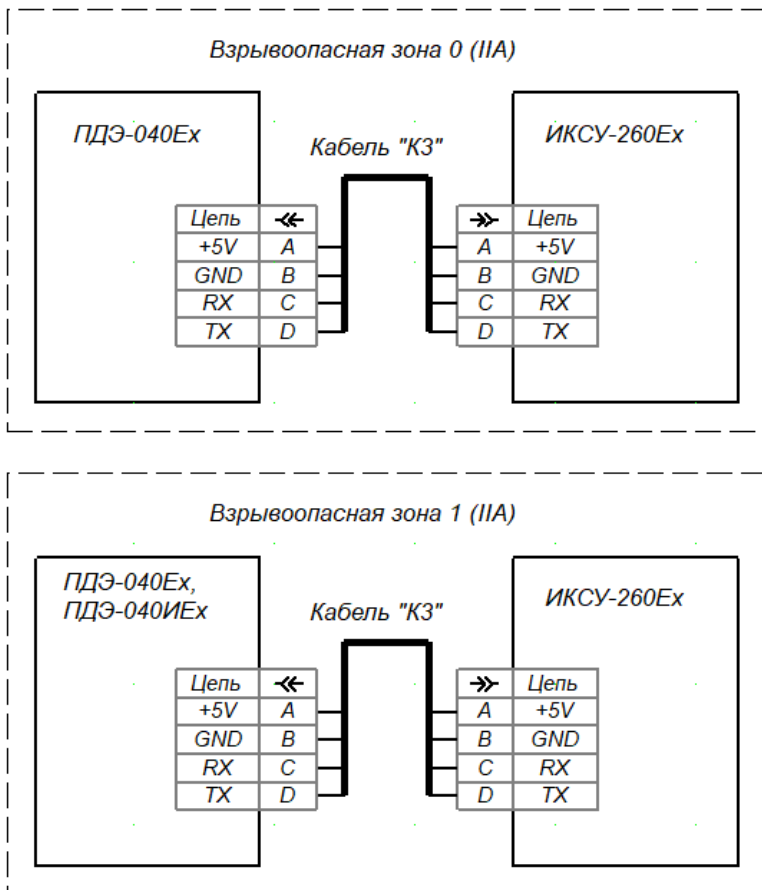
Рисунок Б.4 – Схема электрическая подключений ПДЭ-040Ex, ПДЭ-040IEx к ИКСУ-260Ex
