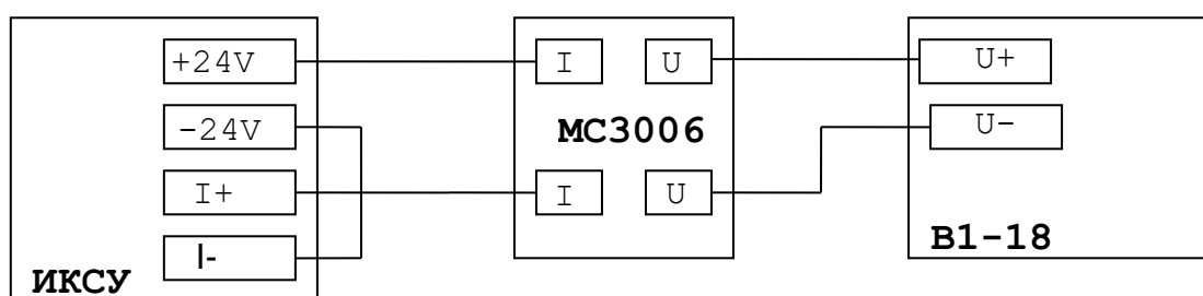
Рисунок 4.4 – Схема проверки ИКСУ-260 в режиме воспроизведения силы постоянного тока
