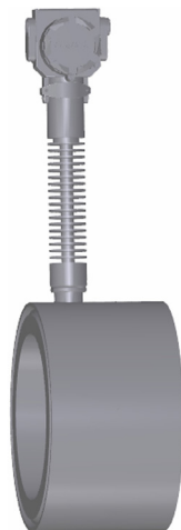
PB DN250-PN100-160-СП-Э-ТР1
