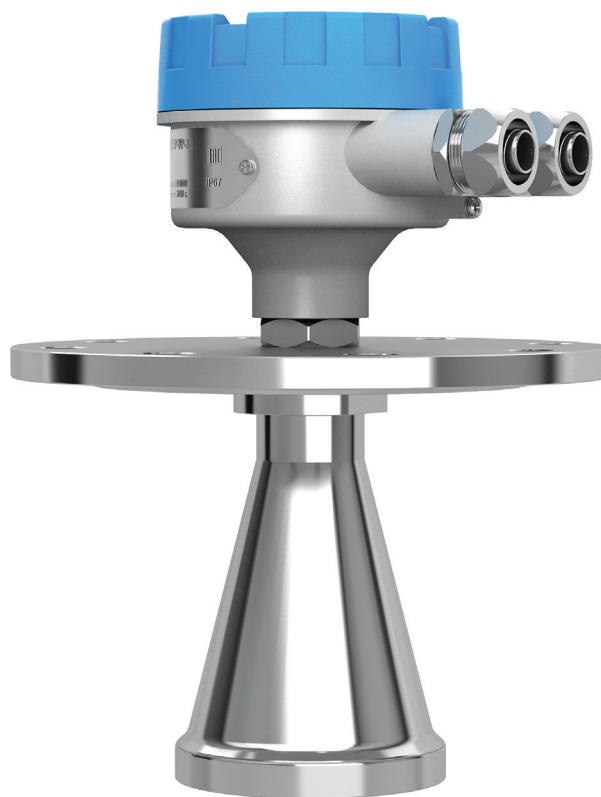
Рис. 1. Радарный уровнемер «ЭЛЕМЕР-УР-31»
