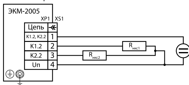
ЭКМ-2005 в корпусе АГ-16 без токового выхода с напряжением питания =24 В или =36 В
