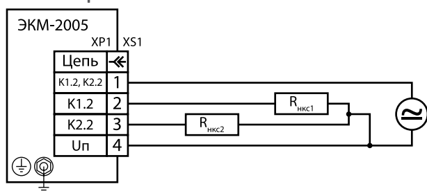
ЭКМ-2005 в корпусе АГ-16 без токового выхода с напряжением питания ~220 В или =220 В
