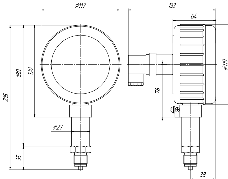
ЭКМ-2005 в корпусе АГ-16И1 (односекционный)
