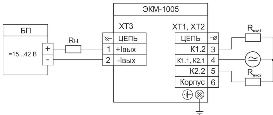
Рисунок 3.3 - Схема электрическая подключений ЭКМ-1005 через кабельный ввод с каналами сигнализации
