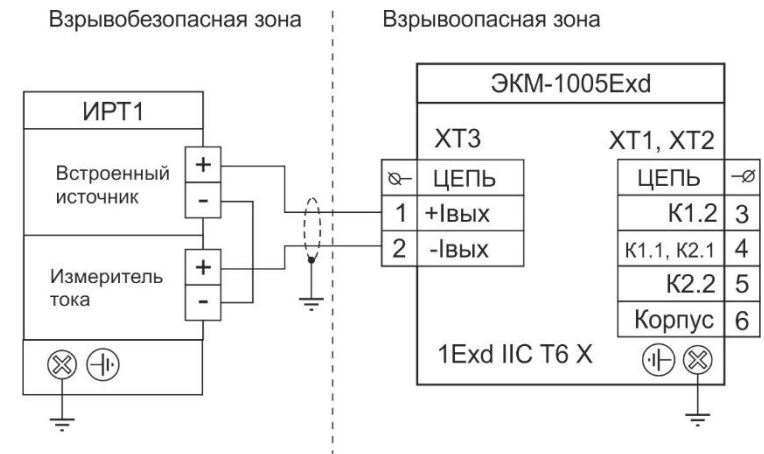
Рисунок 3.6 - Схема электрическая подключений ЭКМ-1005Exd через кабельный ввод без каналов сигнализации к приборам производства НПП «ЭЛЕМЕР»
