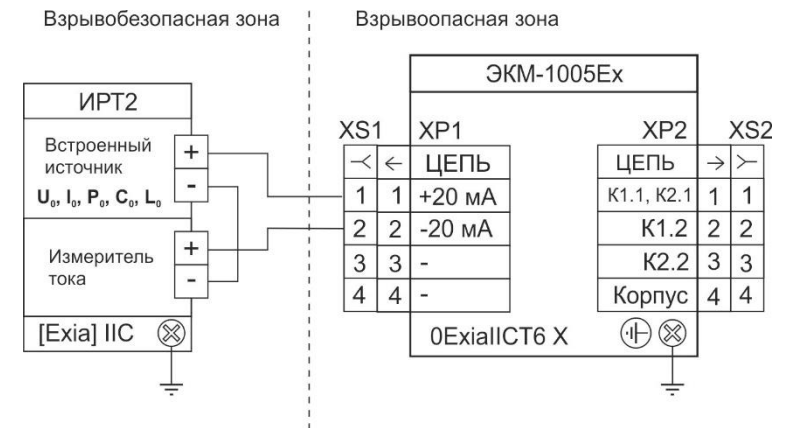
Рисунок 3.8 - Схема электрическая подключений ЭКМ-1005Ex через разъемы GSP 3 M20 (GSP 311) без каналов сигнализации
