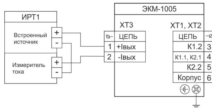
Рисунок 3.2 - Схема электрическая подключений ЭКМ-1005 через кабельный ввод без каналов сигнализации к приборам производства НПП «ЭЛЕМЕР»
