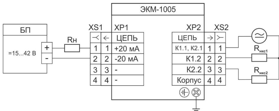
Рисунок 3.3 - Схема электрическая подключений ЭКМ-1005 через кабельный ввод с каналами сигнализации
