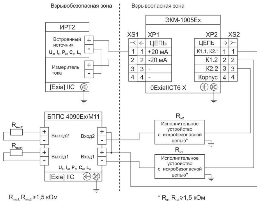
Рисунок 3.9 - Схема электрическая подключений ЭКМ-1005Ex через разъемы GSP 3 M20 (GSP 311) с каналами сигнализации
