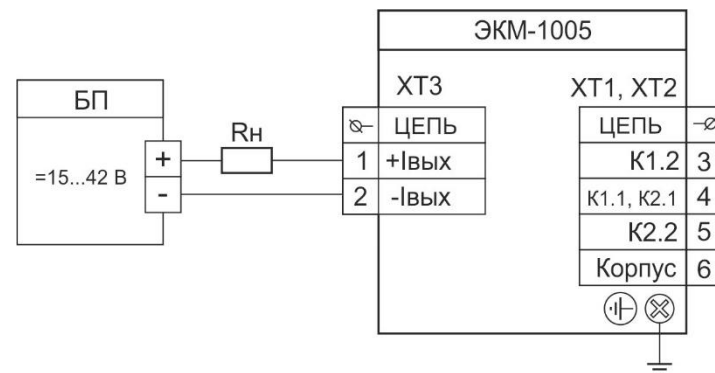
Рисунок 3.1 - Схема электрическая подключений ЭКМ-1005 через кабельный ввод без каналов сигнализации
