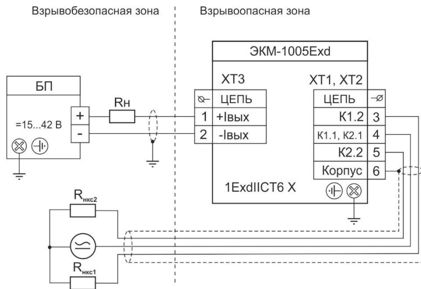
Рисунок 3.7 - Схема электрическая подключений ЭКМ-1005Exd через кабельный ввод с каналами сигнализации
