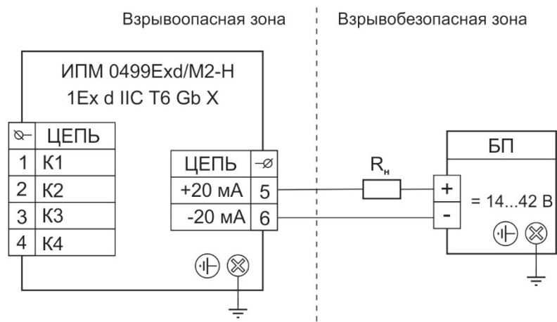
Рисунок Б.4 – Схема электрическая подключений ИПМ 0499Exd/M2-H
