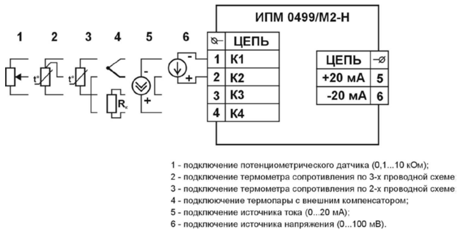
Рисунок Б.1 – Схема электрическая подключений датчиков к ИПМ 0499/М2-Н
