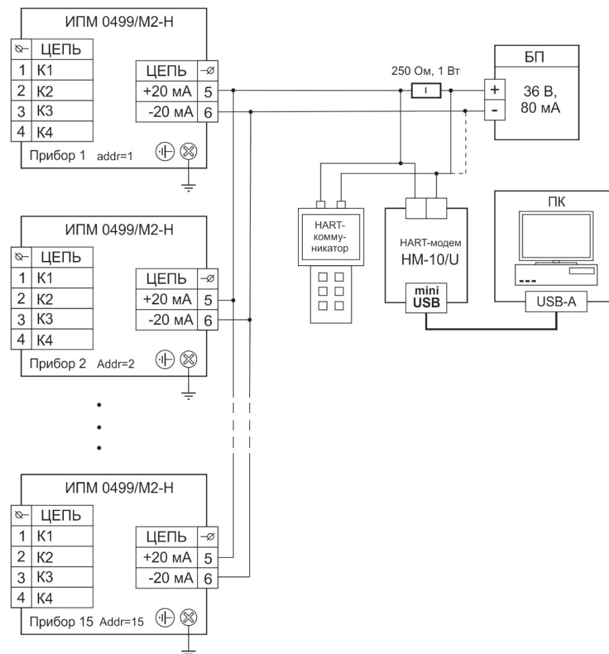
Рисунок Б.6 - Схема электрическая подключений ИПМ по HART-протоколу в сетевом режиме
