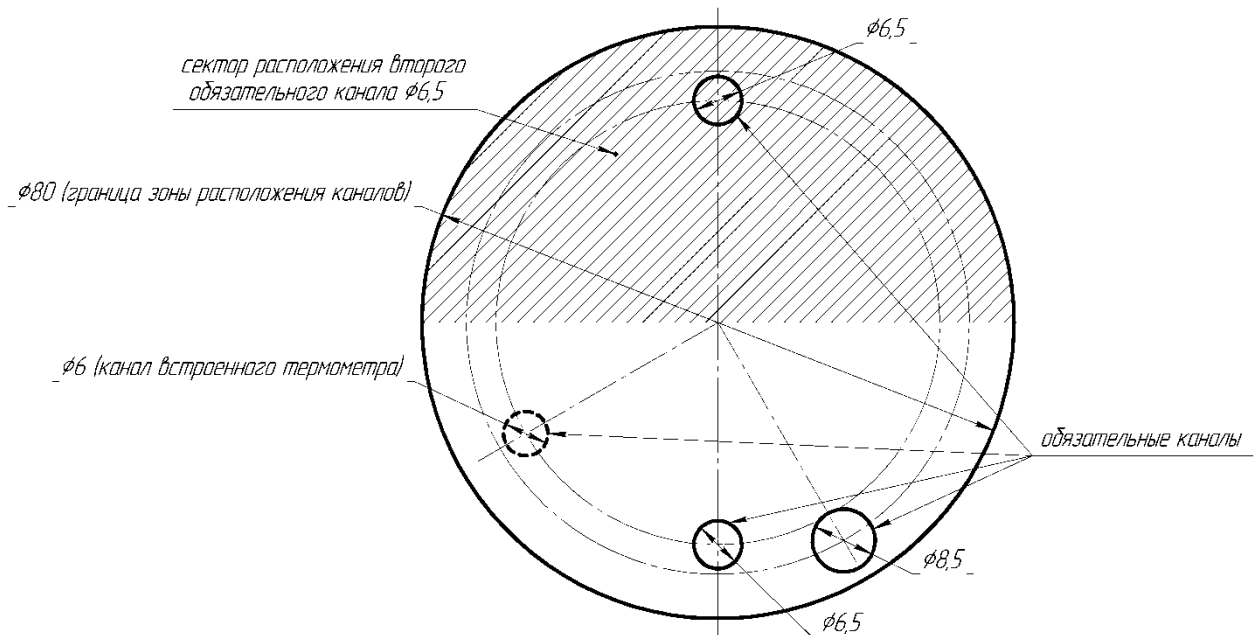
Рисунок А.4 Нестандартный набор каналов в термостатирующем блоке ЭЛЕМЕР-КТ-500/М1*
