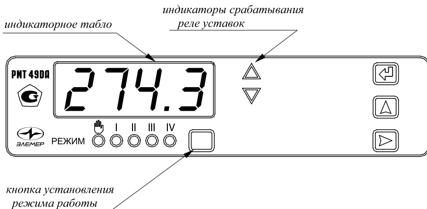
Регистратор многоканальный технологический PMT 49DA/1. Передняя панель
