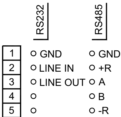
Назначение контактов интерфейсного разъема
