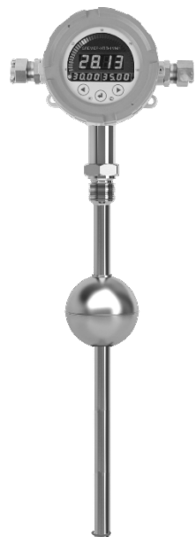
«ЭЛЕМЕР-УПП-11/М1»
