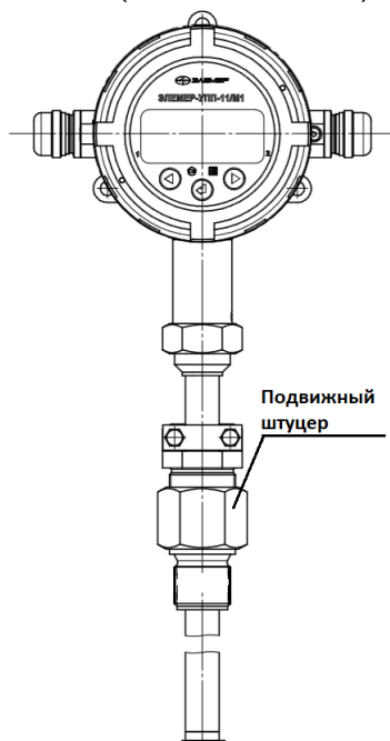
Рисунок В.2 - УПП-11/М1, УПП-11/М1L с подвижным штуце- ром, индекс заказа «ПШ»
