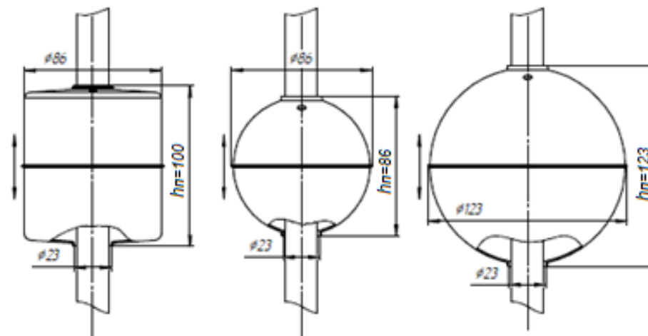
Рисунок А.4 - Размеры поплавков УПП-11/М1, УПП-11/М1L
