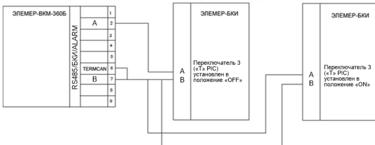
Схема соединений БВ и нескольких БКИ в вычислителях ЭЛЕМЕР-ВКМ-360Б
