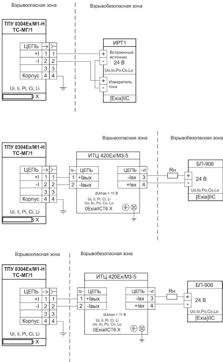
Рисунок А.18 - Схема электрическая подключений ТПУ 0304/М1-Н с ТС-МГ/1 по токовой петле 4-20 мА во взрывоопасной зоне
