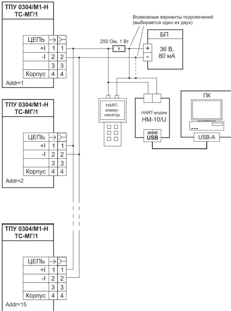
Рисунок А.20 - Схема «многоточечного» (сетевое) подключения ТПУ 0304/М1-Н с ТС-МГ/1 с ТС-МГ/1 по HART-протоколу. (Короткий адрес = 1...15)
