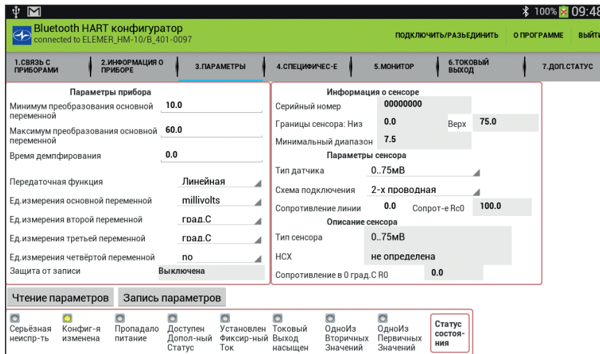
Закладка «Параметры»
