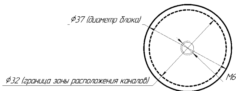
Рисунок Б.2.6 – Эскиз для расположения нестандартного набора каналов в блоке сравнения сменном НБС-КТ-200К/М2 (только для ЭЛЕМЕР-КТ-200К/М2)
