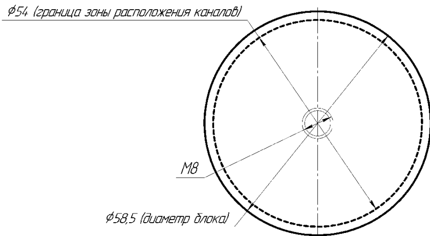
Рисунок Б.5.4 – Эскиз для расположения нестандартного набора каналов в блоке сравнения сменном НБС-КТ-680К
