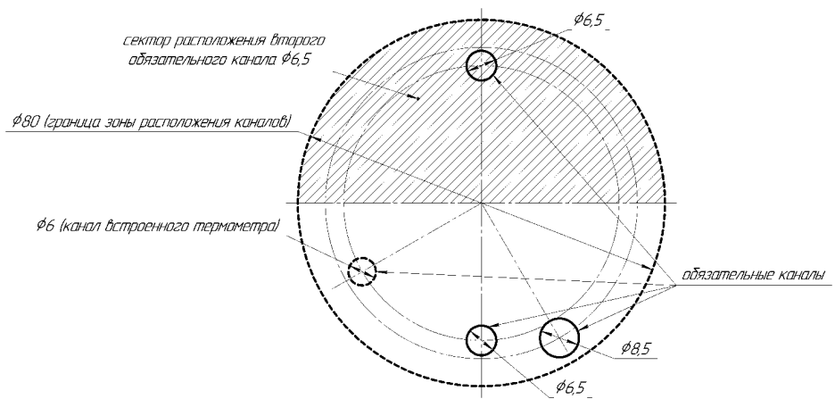
Рисунок Б.3.2 – Эскиз для расположения нестандартного набора каналов (НТБ) в термостатирующем блоке ЭЛЕМЕР-КТ-500К/М1
