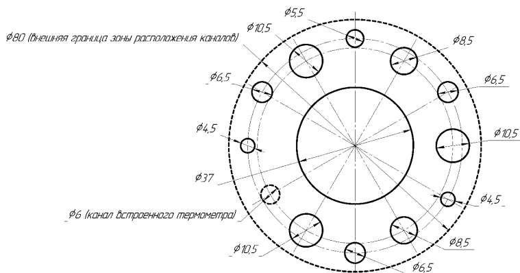
Рисунок Б.4.3 – Расположение стандартного набора каналов (СТБ) в термостатирующем блоке ЭЛЕМЕР-КТ-650К/М2
