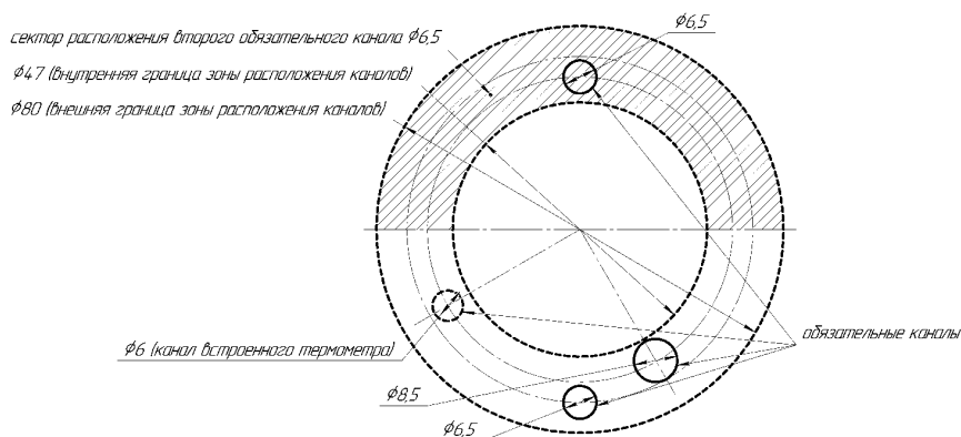
Рисунок Б.3.4 – Эскиз для расположения нестандартного набора каналов (НТБ) в термостатирующем блоке ЭЛЕМЕР-КТ-500К/М2
