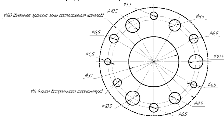
Рисунок Б.3.3 – Расположение стандартного набора каналов (СТБ) в термостатирующем блоке ЭЛЕМЕР-КТ-500К/М2
