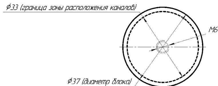
Рисунок Б.3.6 – Эскиз для расположения нестандартного набора каналов в блоке сравнения сменном НБС-КТ-500К/М2 (только для ЭЛЕМЕР-КТ-500К/М2)
