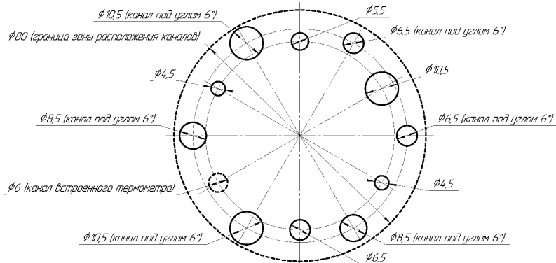
Рисунок Б.4.1 – Расположение стандартного набора каналов (СТБ) в термостатирующем блоке ЭЛЕМЕР-КТ-650К/М1
