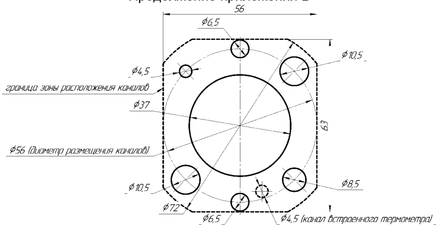
Рисунок Б.2.3 – Расположение стандартного набора каналов (СТБ) в термостатирующем блоке ЭЛЕМЕР-КТ-200К/М2
