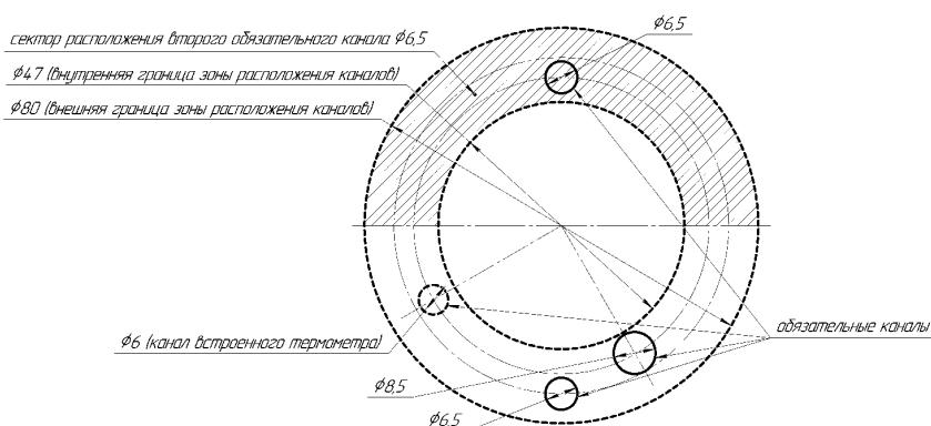
Рисунок Б.4.4 – Эскиз для расположения нестандартного набора каналов (НТБ) в термостатирующем блоке ЭЛЕМЕР-КТ-650К/М2
