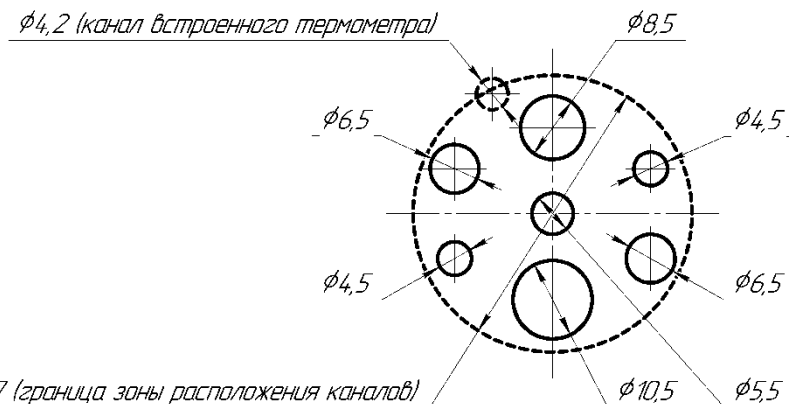
Рисунок Б.1.1 – Расположение стандартного набора каналов (СТБ) в термостатирующем блоке ЭЛЕМЕР-КТ-150К/М1
