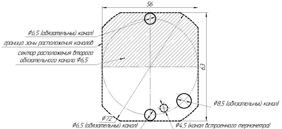
Рисунок Б.2.2 – Эскиз для расположения нестандартного набора каналов (НТБ) в термостатирующем блоке ЭЛЕМЕР-КТ-200К/М1
