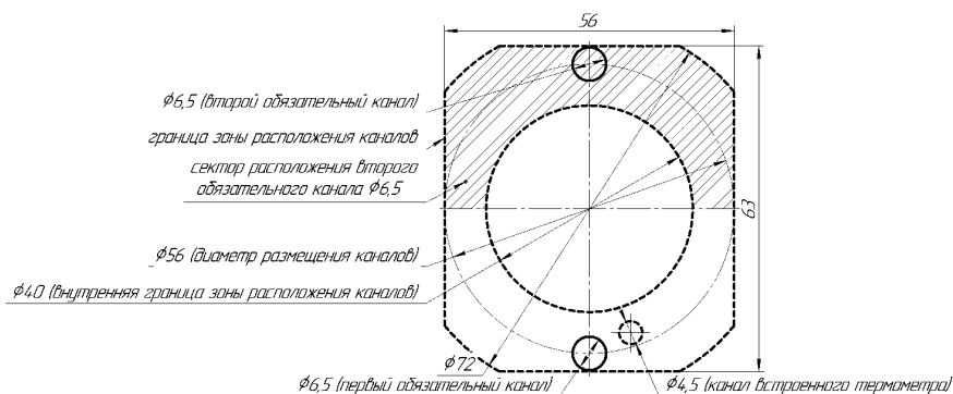
Рисунок Б.2.4 – Эскиз для расположения нестандартного набора каналов (НТБ) в термостатирующем блоке ЭЛЕМЕР-КТ-200К/М2
