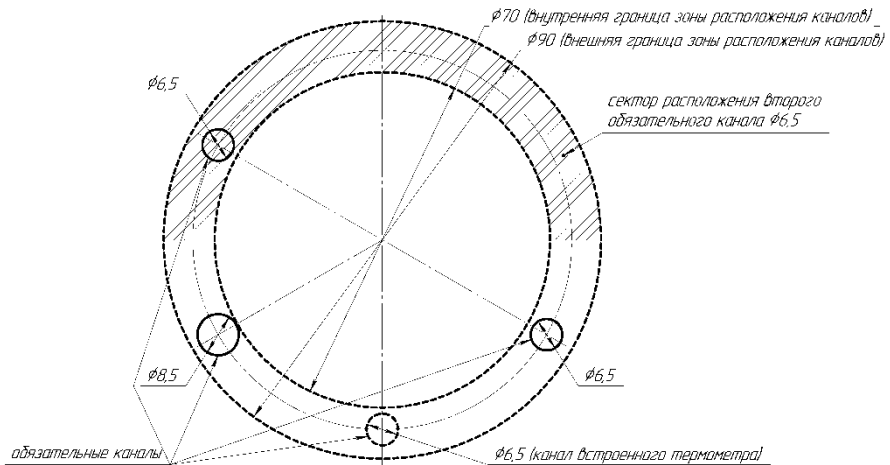
Рисунок Б.5.2 – Эскиз для расположения нестандартного набора каналов (НТБ) в термостатирующем блоке
