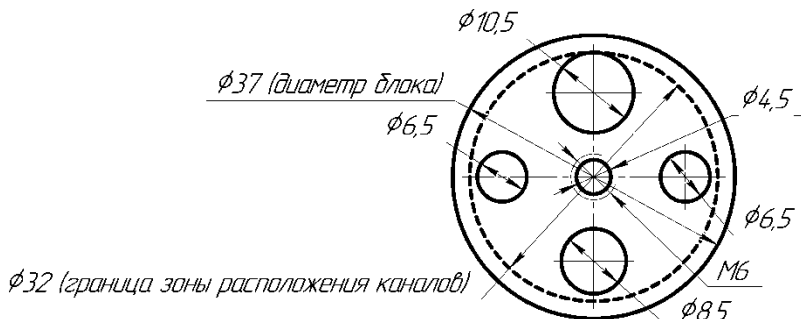
Рисунок Б.2.5 – Расположение стандартного набора каналов в блоке сравнения сменном СБС-КТ-200К/М2 (только для ЭЛЕМЕР-КТ-200К/М2)
