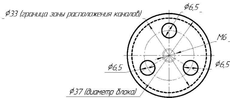
Рисунок Б.4.5 – Расположение стандартного набора каналов в блоке сравнения сменном СБС-КТ-650К/М2 (только для ЭЛЕМЕР-КТ-650К/М2)
