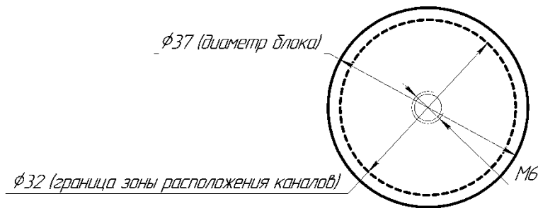
Рисунок Б.1.5 – Эскиз для расположения нестандартного набора каналов в блоке сравнения сменном НБС-КТ-150К/М2 (только для ЭЛЕМЕР-КТ-150К/М2)
