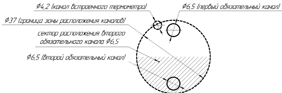
Рисунок Б.1.2 – Эскиз для расположения нестандартного набора каналов (НТБ) в термостатирующем блоке ЭЛЕМЕР-КТ-150К/М1
