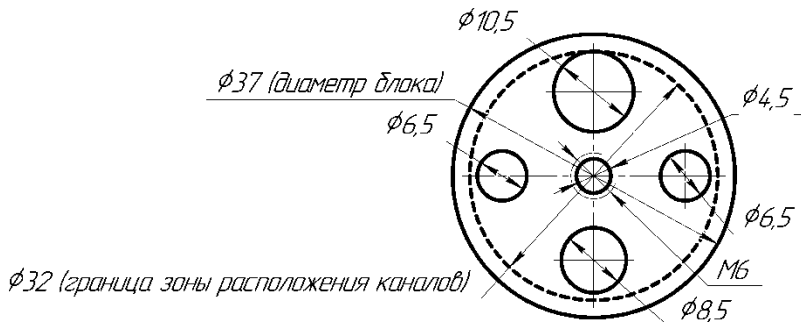
Рисунок Б.1.4 – Расположение стандартного набора каналов в блоке сравнения сменном СБС-КТ-150К/М2 (только для ЭЛЕМЕР-КТ-150К/М2)
