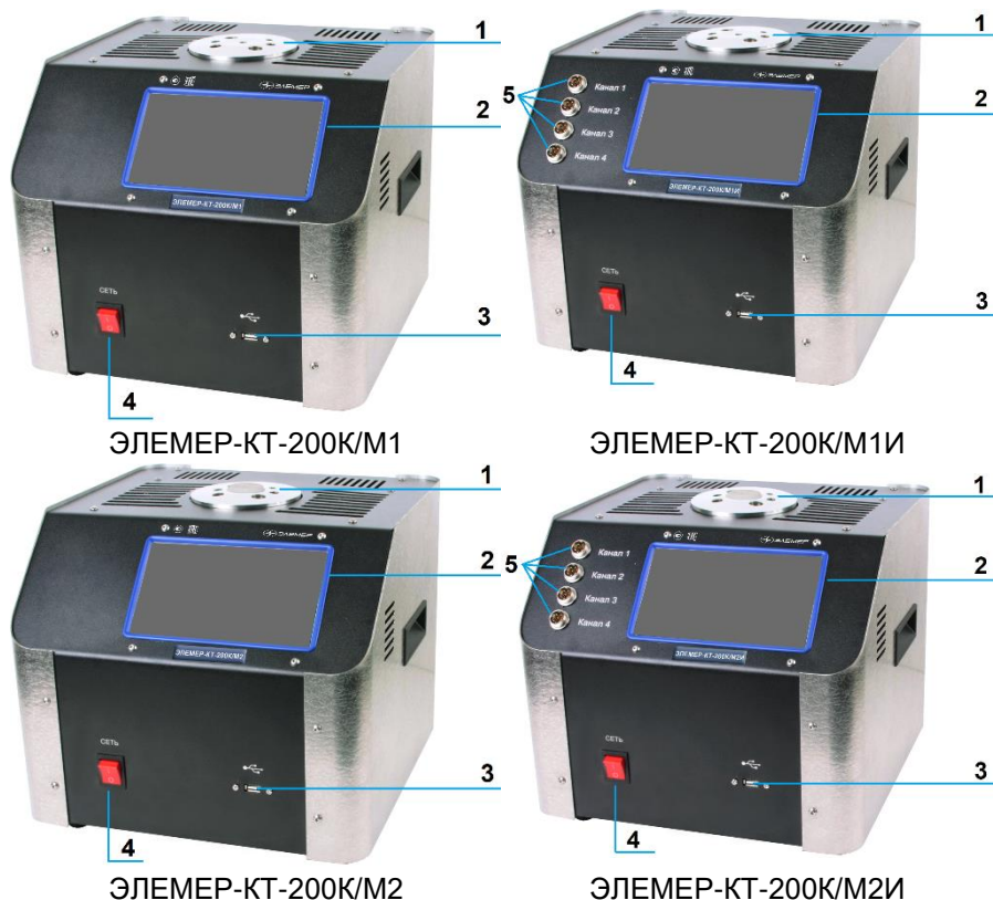
Рисунок 5.1 – Общий вид КТ-150К/М1, КТ-150К/М1И, КТ-150К/М2, КТ-150К/М2И, КТ-200К/М1, КТ-200К/М1И, КТ-200К/М2, КТ-200К/М2И
