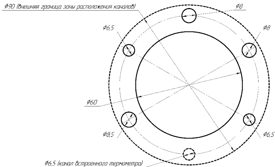
Рисунок Б.5.1 – Расположение стандартного набора каналов (СТБ) в термостатирующем блоке
