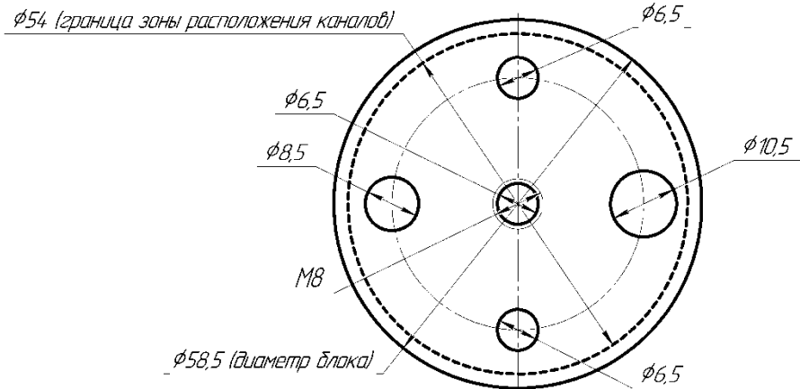
Рисунок Б.5.3 – Расположение стандартного набора каналов в блоке сравнения сменном СБС-КТ-680К
