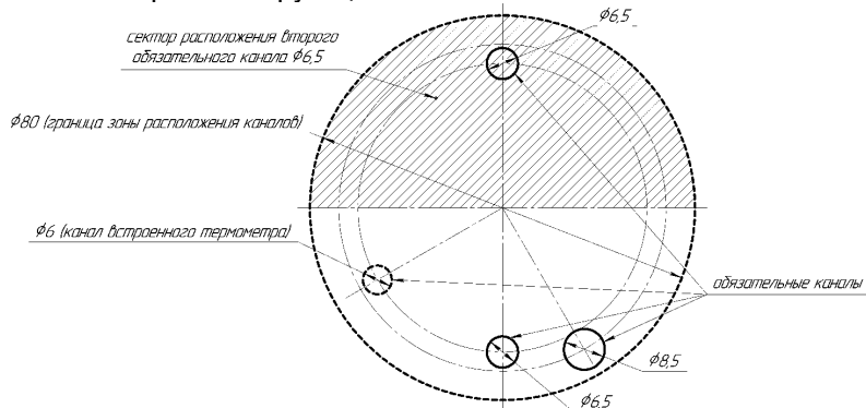
Рисунок Б.4.2 – Эскиз для расположения нестандартного набора каналов (НТБ) в термостатирующем блоке ЭЛЕМЕР-КТ-650К/М1
