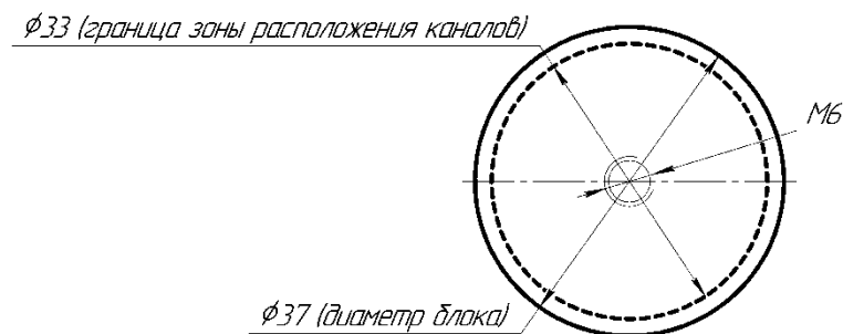
Рисунок Б.4.6 – Эскиз для расположения нестандартного набора каналов в блоке сравнения сменном НБС-КТ-650К/М2 (только для ЭЛЕМЕР-КТ-650К/М2)
