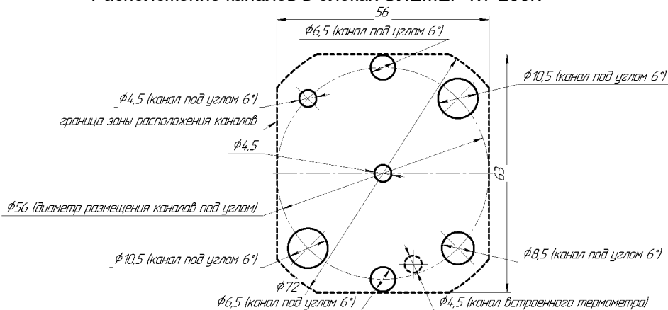
Рисунок Б.2.1 – Расположение стандартного набора каналов (СТБ) в термостатирующем блоке ЭЛЕМЕР-КТ-200К/М1
