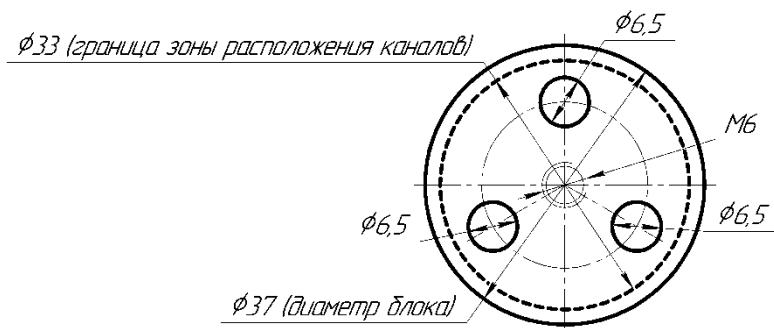
Рисунок Б.3.5 – Расположение стандартного набора каналов в блоке сравнения сменном СБС-КТ-500К/М2 (только для ЭЛЕМЕР-КТ-500К/М2)
