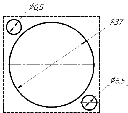
Рисунок Б.1.3 – Расположение стандартного набора каналов (СТБ) в термостатирующем блоке ЭЛЕМЕР-КТ-150К/М2
