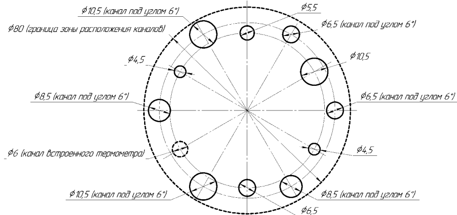
Рисунок Б.3.1 – Расположение стандартного набора каналов (СТБ) в термостатирующем блоке ЭЛЕМЕР-КТ-500К/М1
