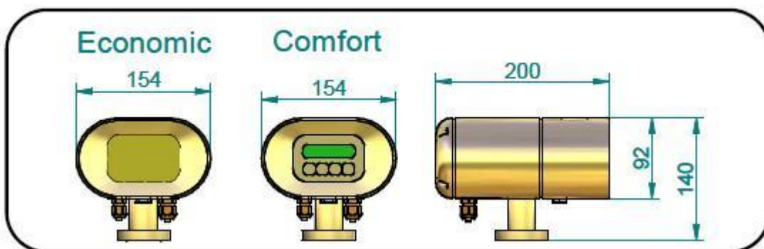
Габаритные размеры для монтажа блока электроники компактном исполнении
