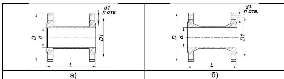
Рисунок Ж.4 – Вставки монтажные ЭЛЕМЕР-РВ (тип присоединения к процессу «сэндвич»)
