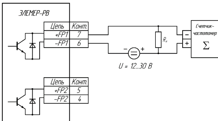
Рисунок А.3 – Схема электрическая подключений электронного счетчика-частотомера к дискретным выходам ЭЛЕМЕР-PB. R_H = 1 \text{ кОм} . Подключение к цепям «+FP2» и «-FP2» аналогичное
