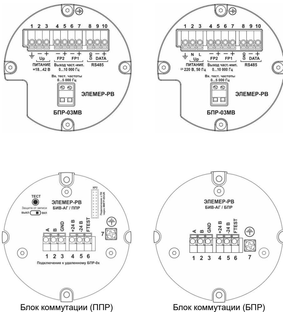
Рисунок 2.4 – Модуль подключений расходомера
