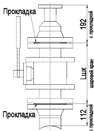
Рисунок 3.23 – Конструктивный размер расходомера С (рисунок 3.22)
