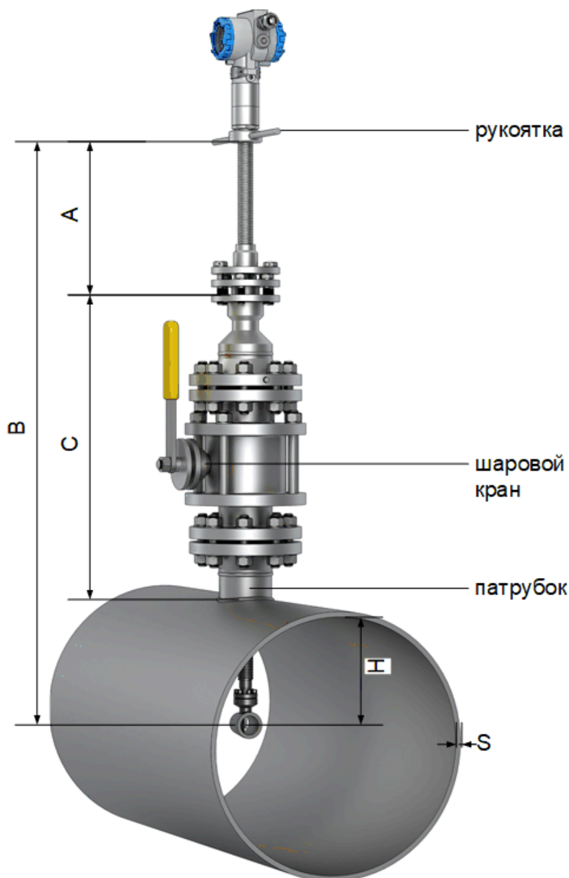
Рисунок 3.22 – Внешний вид расходомера (тип присоединения к процессу «зондовый с лубрикаторм»), установленного в трубопровод
