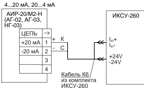
Рисунок 3.2 – Схема электрическая подключений.
