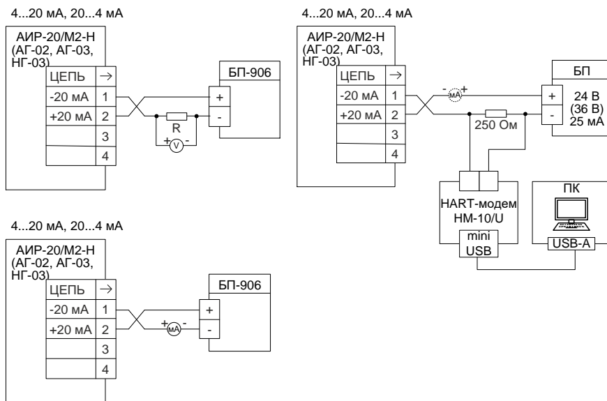
Рисунок 3.2 – Схема электрическая подключений.
