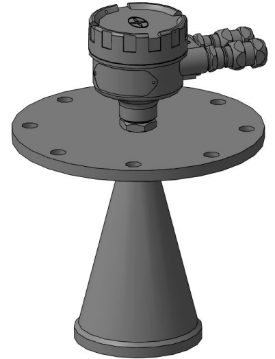
ЭЛЕМЕР-УР-31-M3-DN150
