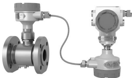
раздельное исполнение фланцевое с БПР без индикации
