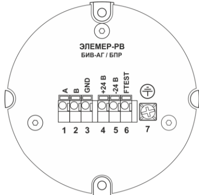
Блок коммутации (БПР)
