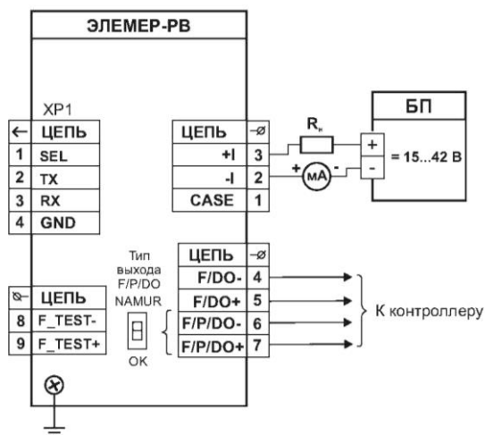
Рисунок А.1 – Схема электрическая подключений ЭЛЕМЕР-РВ по токовой петле
