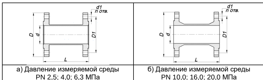
Рисунок Е.4 – Вставки монтажные ЭЛЕМЕР-РВ (тип присоединения к процессу «сэндвич»)
