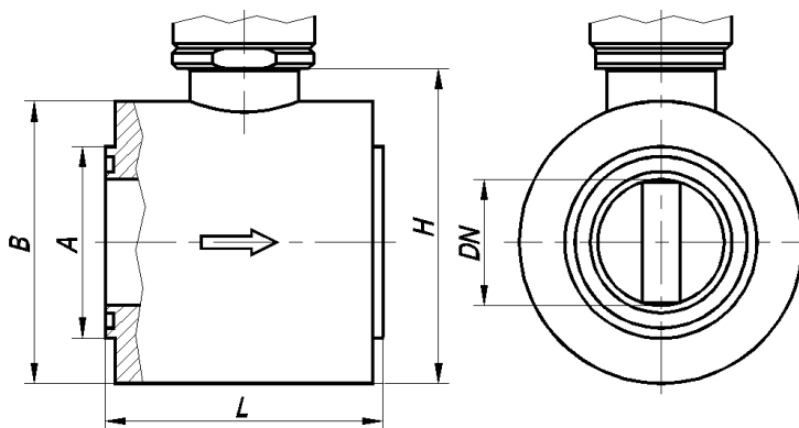
Рисунок Б.6 – Компактное исполнение расходомера (тип присоединения к процессу «сэндвич», тип 1, номинальное давление среды 2,5; 4,0; 6,3; 10,0; 16,0 МПа)
