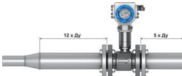
Рисунок 3.4 – Минимальные прямолинейные участки при расширении трубопровода перед расходомером
