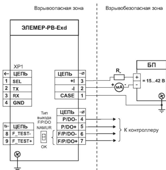
Рисунок А.2 – Схема электрическая подключений ЭЛЕМЕР-РВ-Exd по токовой петле во взрывоопасной зоне
