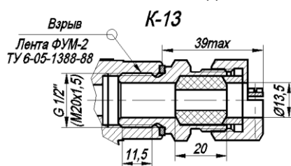
Рисунок Б.12 – Чертеж средств взрывозащиты (компактное исполнение с БПР-02/М2)
