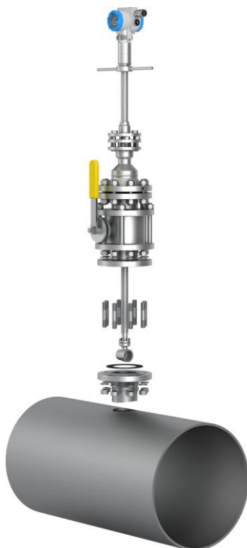
Рисунок 3.25 – Монтаж расходомера (тип присоединения к процессу «зондовый с лубрикатом»)
