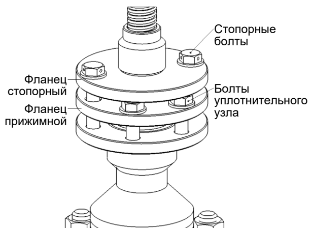
Рисунок 3.26 – Внешний вид уплотнительного узла расходомера (тип присоединения к процессу «зондовый с лубрикатом»)
