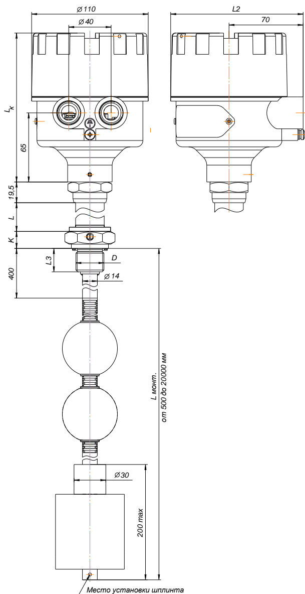
Рисунок Б.4 – ЭЛЕМЕР-УПМ-51/МЗИ с гибким измерительным элементом
