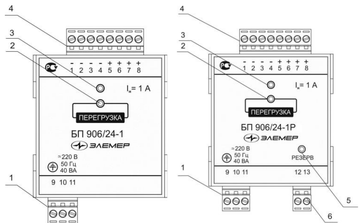
Передняя панель БП 906/24-1
