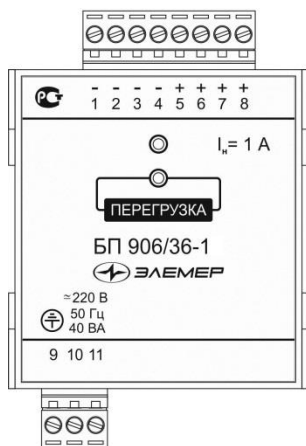
Передняя панель БП 906/36-1
