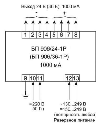
Схема подключения БП 906/24(36)-1P
