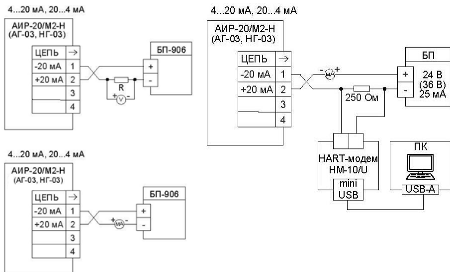
Рисунок 3.2 - Схема электрическая подключений. Вариант с полярностью подключения питания «К1+»
