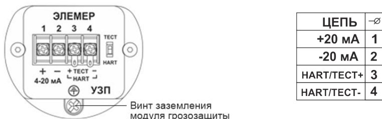
Рисунок 2.4 - Внешний вид коммутационной платы и функциональное расположение контактов для корпуса АГ-03, НГ-03 (АИР-20/М2-Н-ГС со встроенным модулем грозозащиты)
